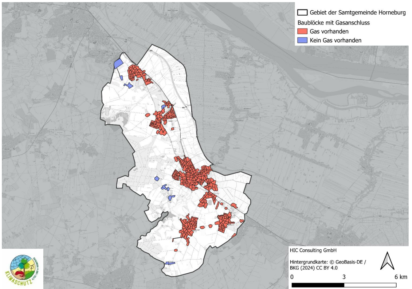
Abbildung 3-12: Versorgungsbereich der Gasnetze / Lage des Gasnetzes in Horneburg
